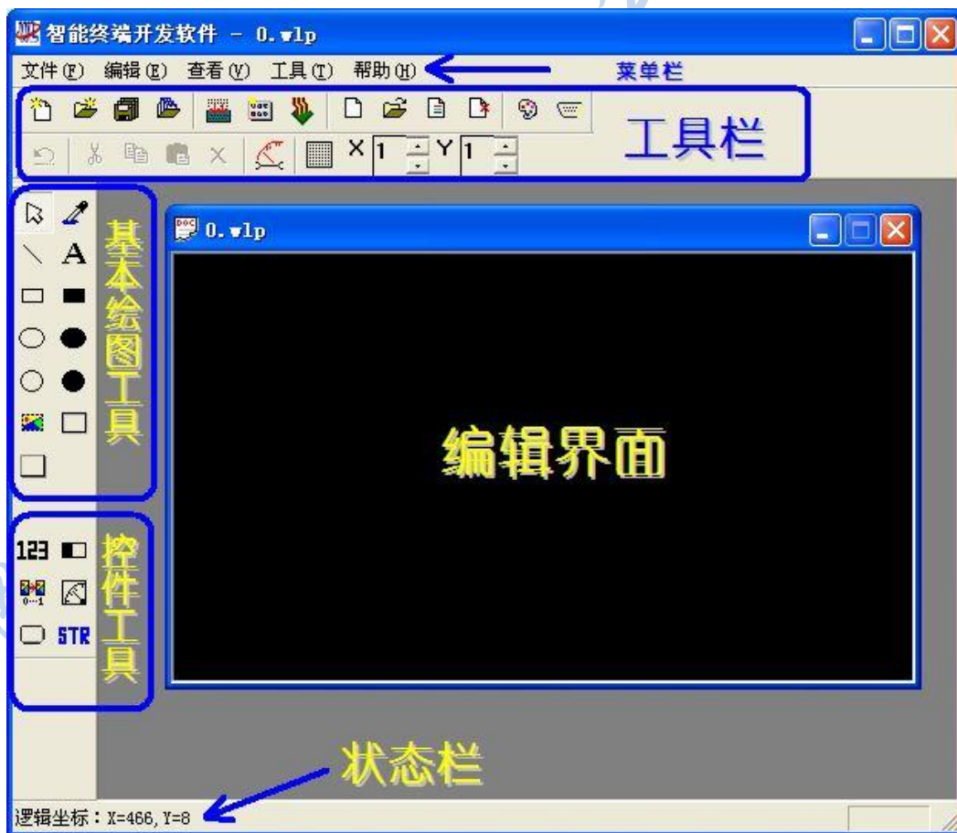
软件整体界面 图 1
